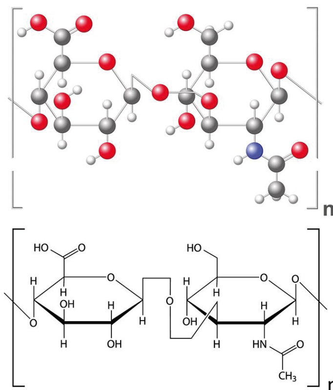
Struttura chimica dell'Acido ialuronico
